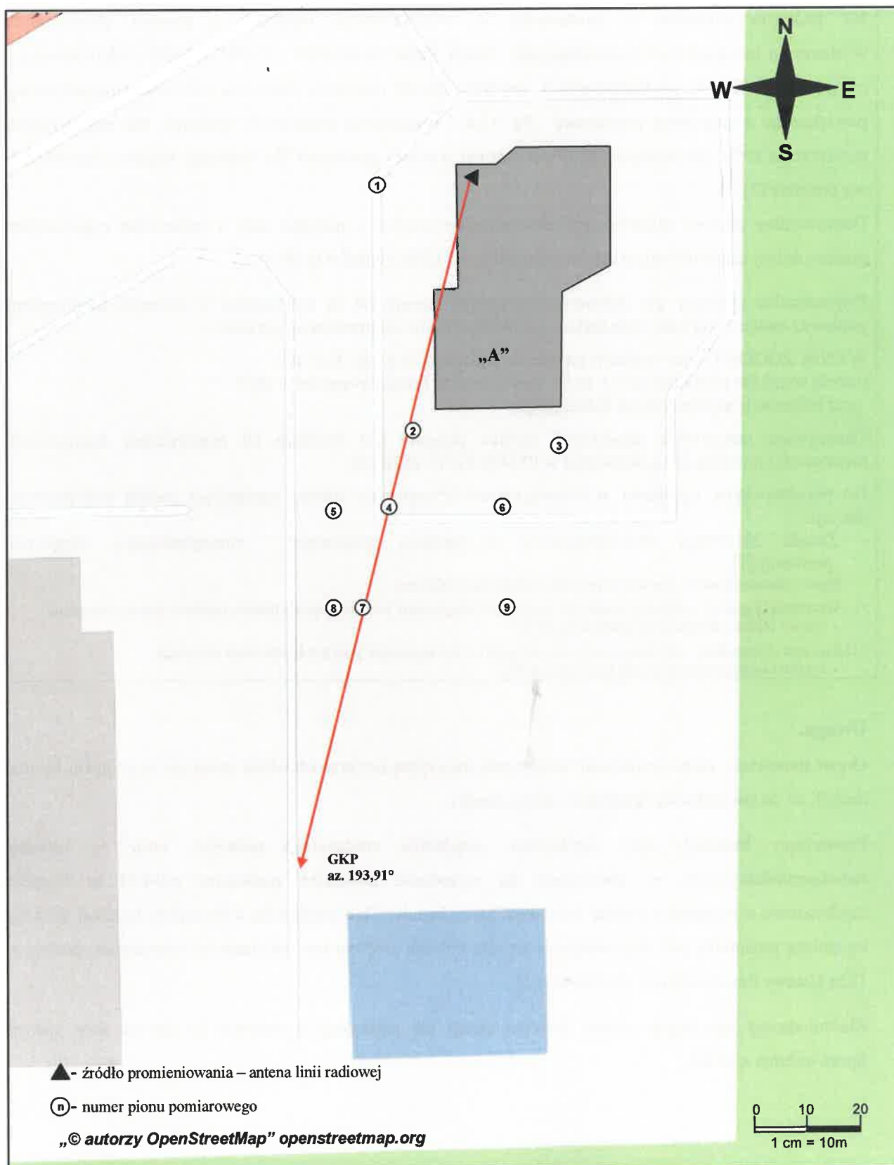
Rys. 1. Usytuowanie punktów i pionów pomiarowych w otoczeniu instalacji radiokomunikacyjnej Stacja Netia DABKB001-DABKM00004 Karpin, ul. Białostocka 8
